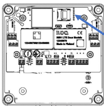
N501 Türmodul
